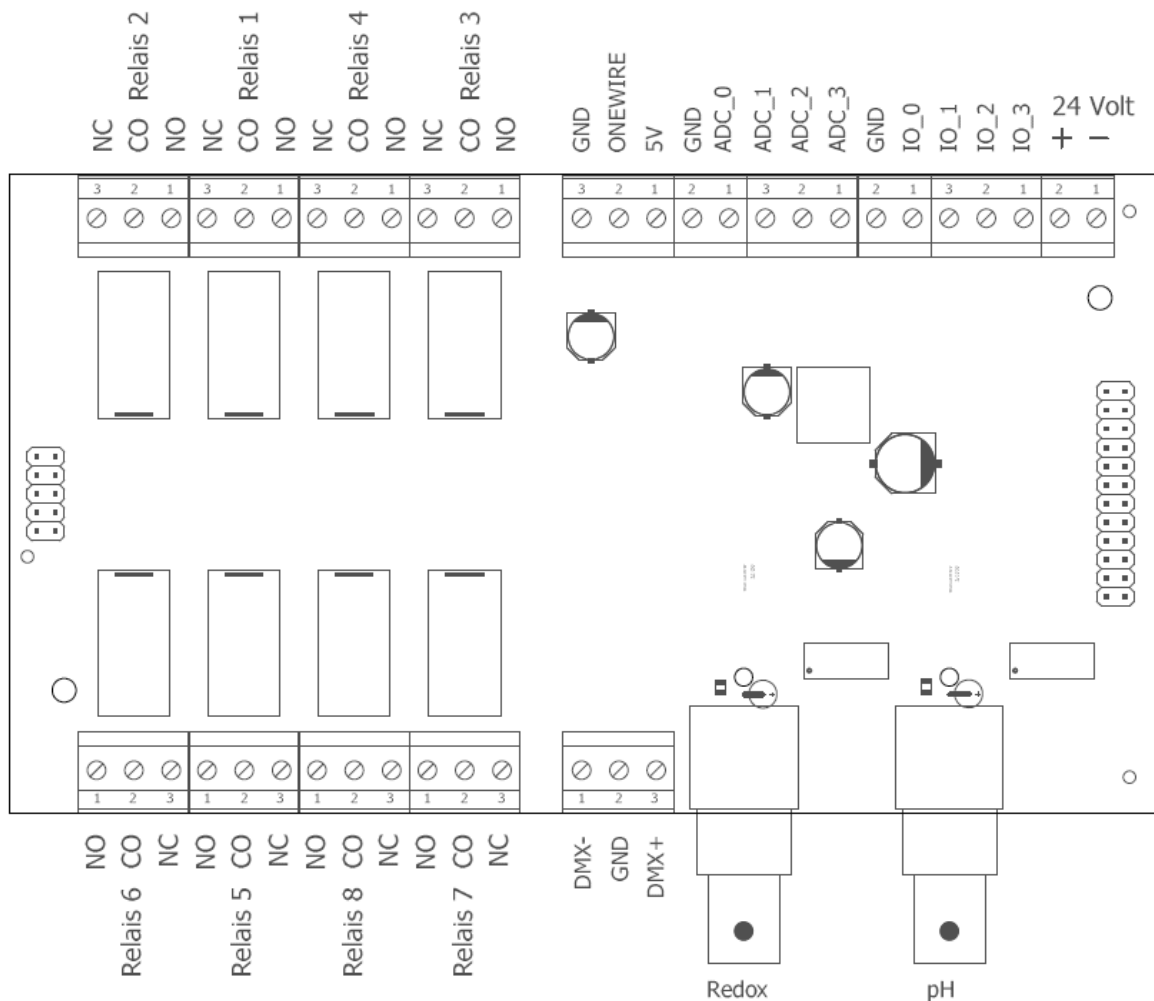
Abbildung 1: Anschlüsse der Steuerung
