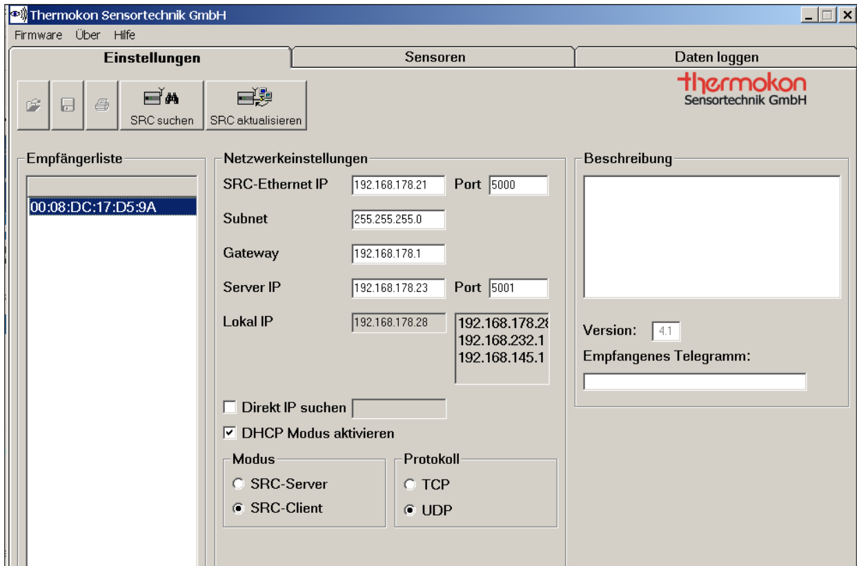
Abbildung 71: Konfiguration STC Thermokon Gateway
