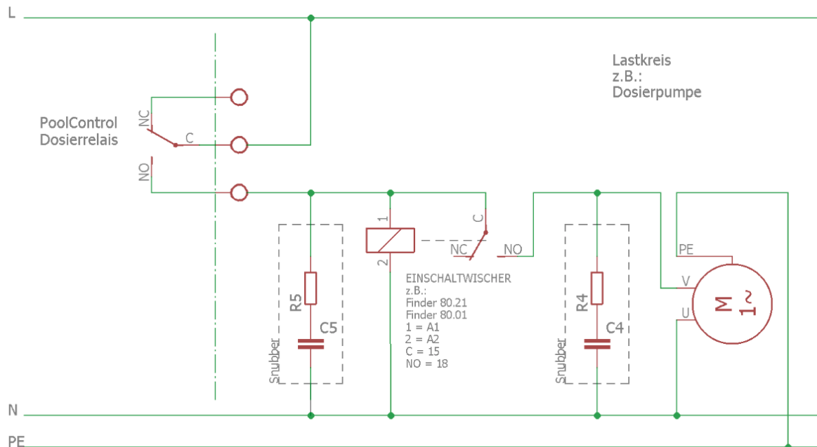
Abbildung 61: 230V Variante
