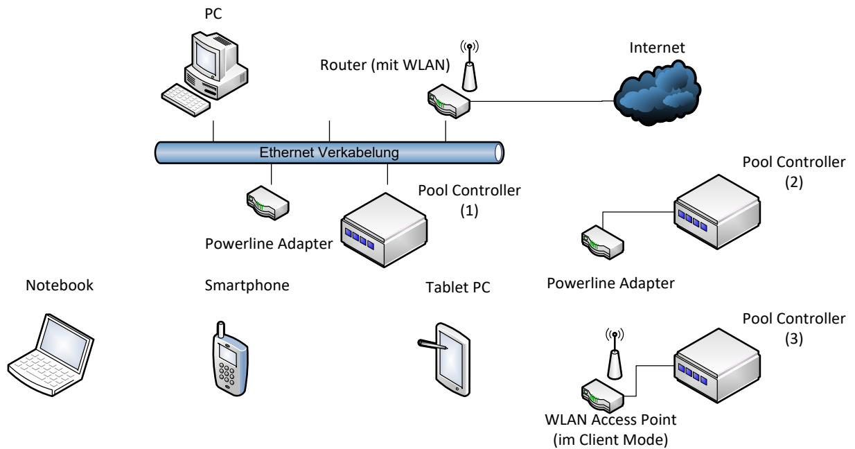
Abbildung 72: Möglichkeiten der Netzwerktopologie
