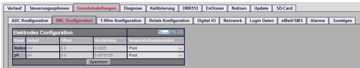
Abbildung 29: BNC Konfiguration
