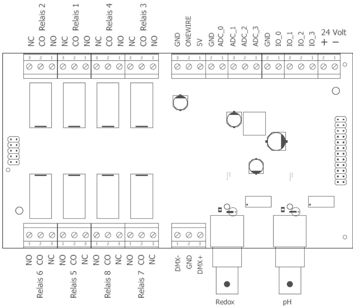
Abbildung 60: Anschlussplan ProCon.IP
