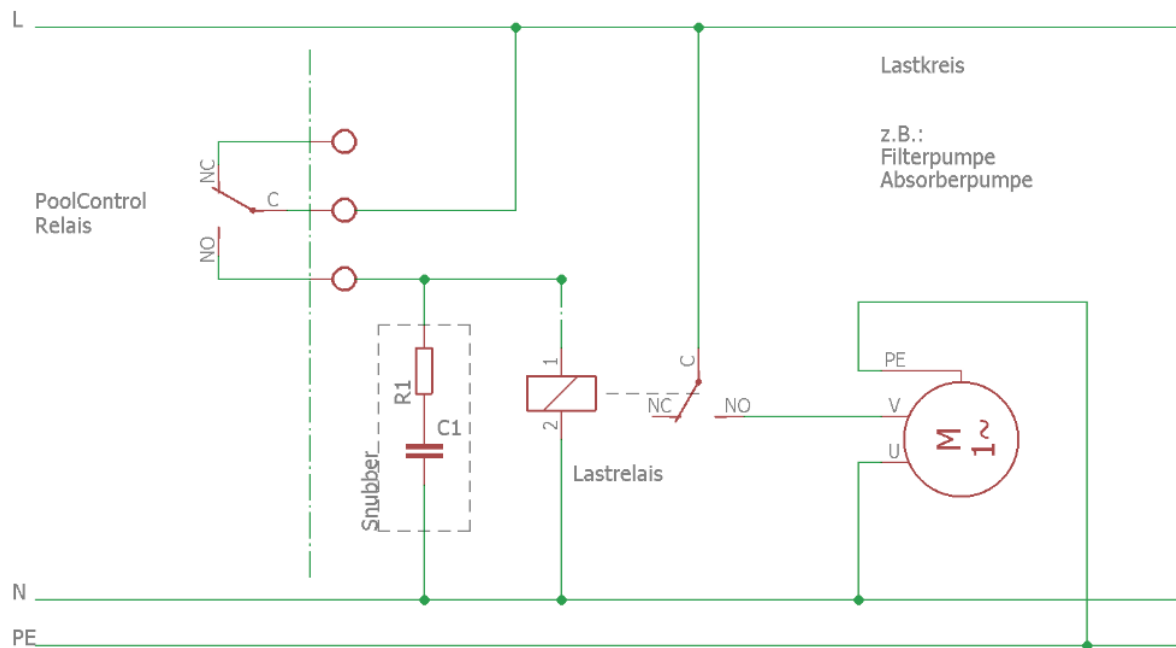
Abbildung 62: 230V Variante
