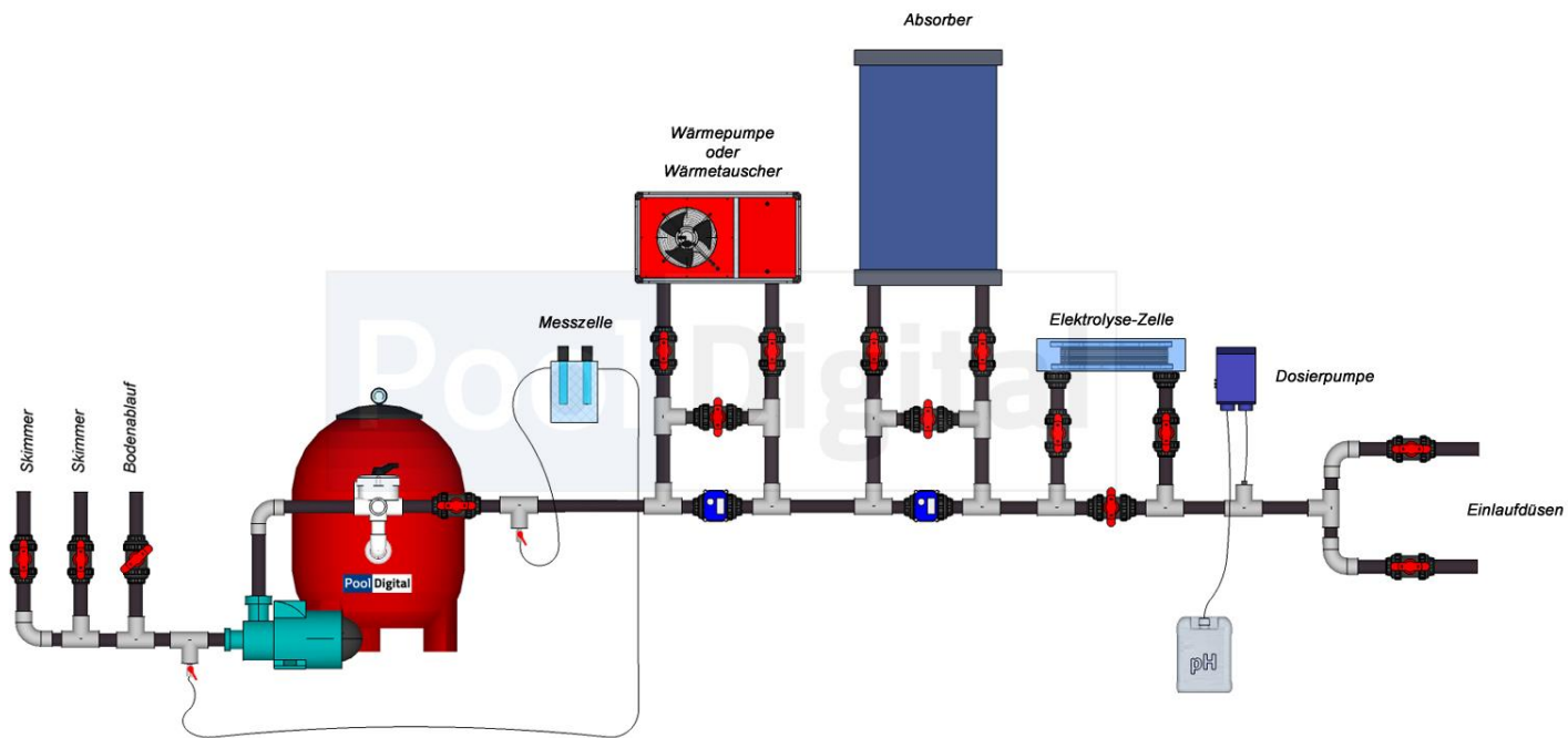
Abbildung 74: Verrohrungsschema bei Salz-Elektrolyse
