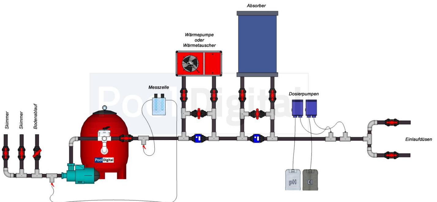
Abbildung 73: Verrohrungsschema Flüssigdosierung
